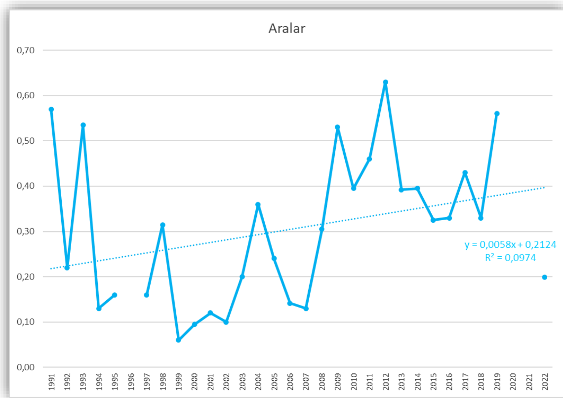
Figura 10 Evolución de la liebre europea en la sierra de Aralar en el periodo 1991-2022. Se indica la abundancia media anual (IKA) y su recta de regresión.
