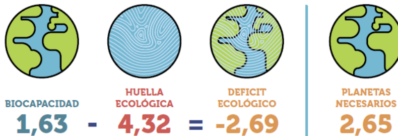
Figura 3. Euskadiko aztarna ekologikoaren emaitza nagusiak
