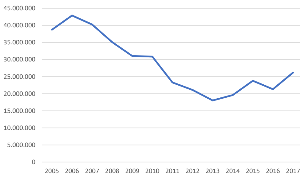
Figura 2. Materialen etxeko kontsumoa EAEn, 2005-2017 1 (tonak)
